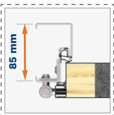
Ościeżnica PERFOTHERM 50*
