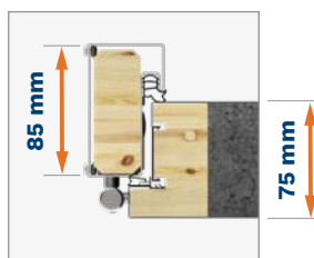
Ościeżnica DUOTHERM 75
