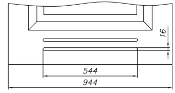
skrzydło „90” ze szczeliną wentylacyjną
