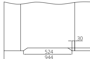
skrzydło „90” z podcięciem wentylacyjnym
