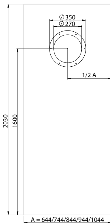
Budowa skrzydła Bulaj przylgowego
