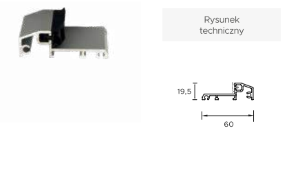
Opaska z ościeżnicą regulowaną Iron
