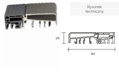
Próg PVC z uszczelką Premium
