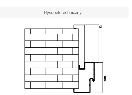
Portal z ościeżnicą wewnętrzną Iron
