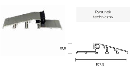
Próg aluminiowy z uszczelką Premium, Normal, Protect, Iron do ościeżnicy "9" (kątovej), "11" (wewnętrznej)
